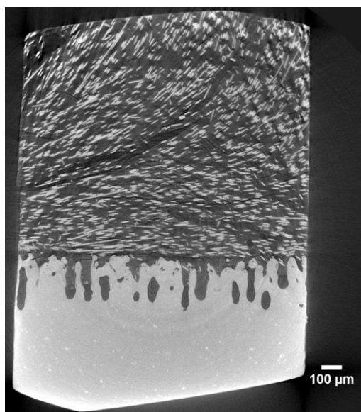
図 1 金属樹脂接合試験片の X 線 CT 画像
