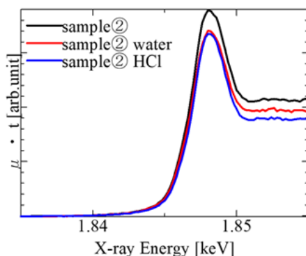
Fig.1 蒸留水及び塩酸洗浄した燃焼灰試料の XANES スペクトル(Ca 近傍)
