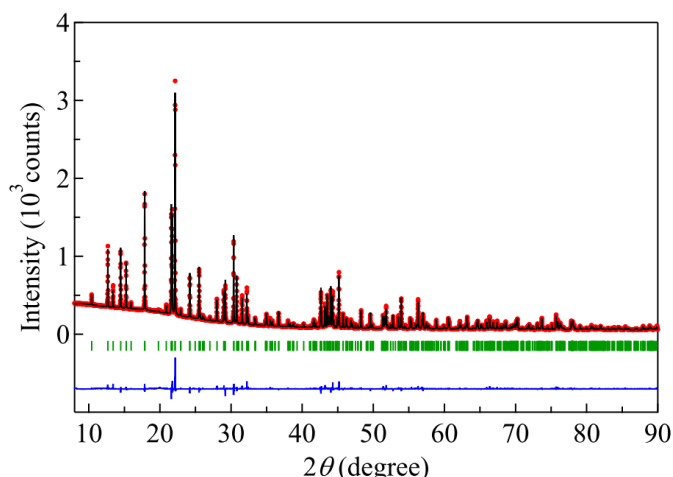
Fig.1 XRD パターンおよび Rietveld 解析結果.
