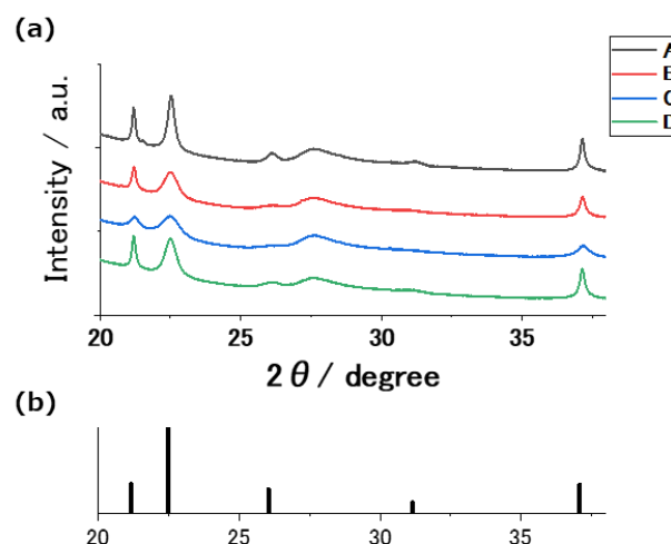
Fig. 1 (a) 条件A-Cで得られた電極材料の粉末X線解析 (b) \text{Li}_2\text{O}_2 のBragg position
